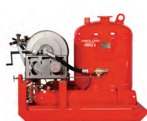
Автоматическая сухая химия Система порошкового тушения
